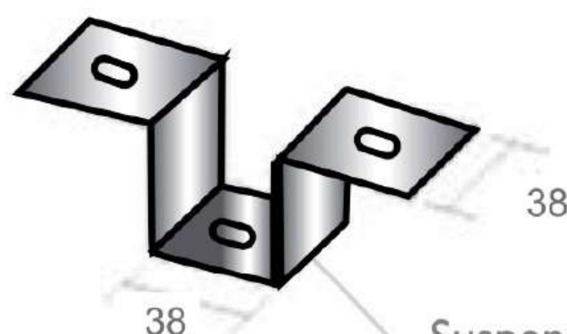
Suspensão p/ Tirante ref: MG 821
