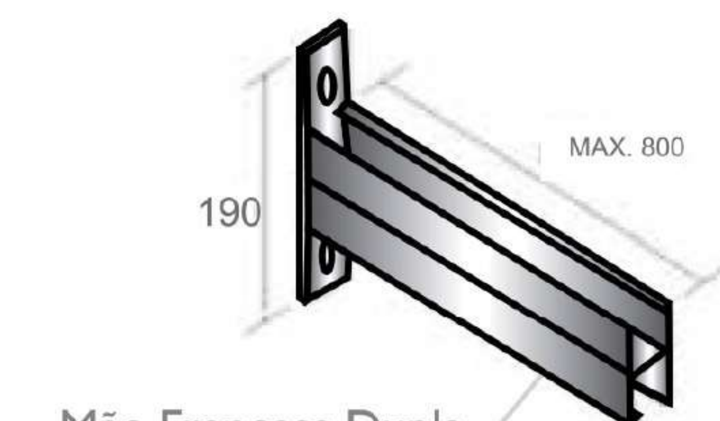
Mão Francesa Dupla 38x38 ref: MG 815
